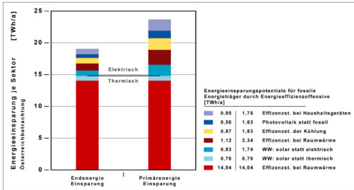
Grafik: Energieeinsparpotentiale Gaskraftwerksneubau versus Energieeffizienz Offensive
