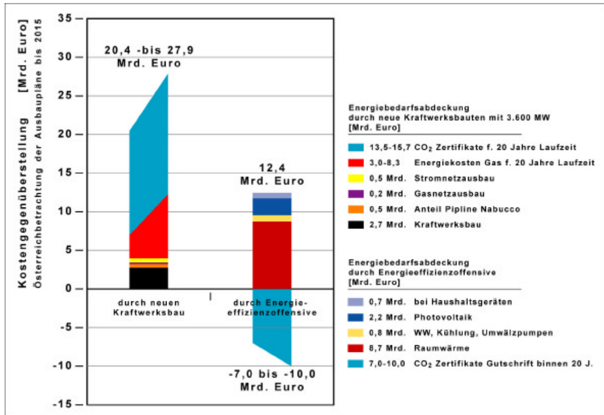
Grafik: Kostengegenüberstellung Gaskraftwerksneubau versus Energieeffizienz Offensive Quelle: IG Passivhaus Österreich, www.igpassivhaus.at
